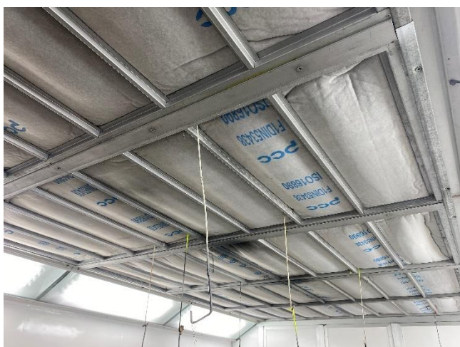
Foto 7 – Filtros de entrada de ar na cabine.
